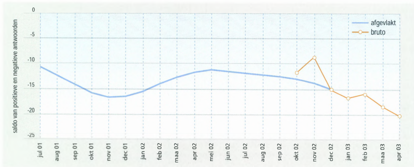
Figuur 2 Synthetische conjunctuurcurve voor West-Vlaanderen
