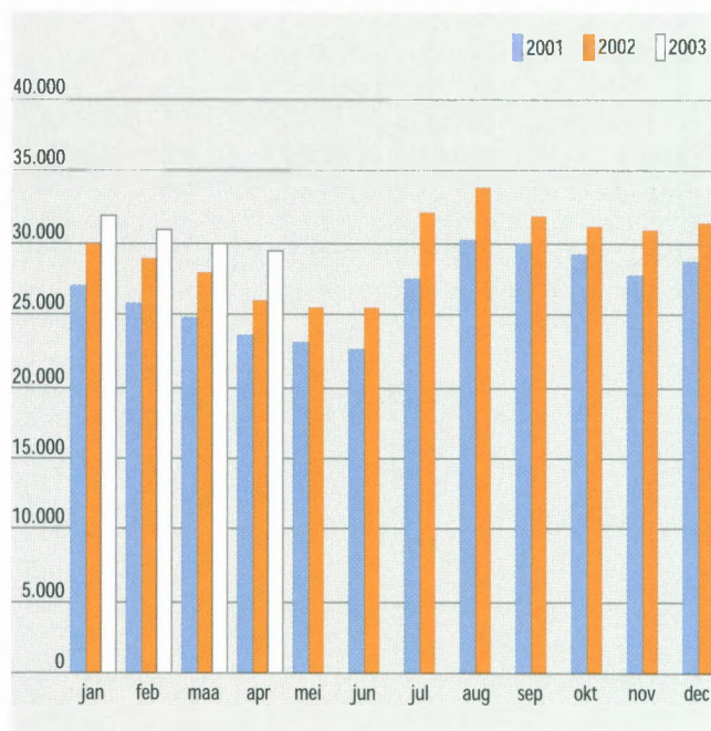
Figuur 1 Evolutie van het aantal niet-werkende werkzoekenden in West-Vlaanderen
