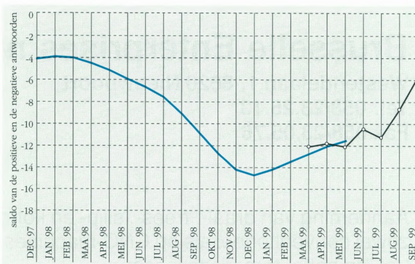
Figuur 3 Synthetische conjunctuurcurve voor West-Vlaanderen, december 1997 - september 1999
