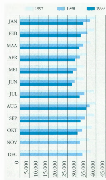
Figuur 1 Evolutie van het aantal niet-werkende werkzoekenden in Vlaanderen
